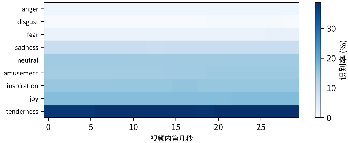
⑨⑫ FACED→讲述 (n=118) · 零样本 · 版本B 总体 12.50% · 恒定 97.9% · 波动 0.4
