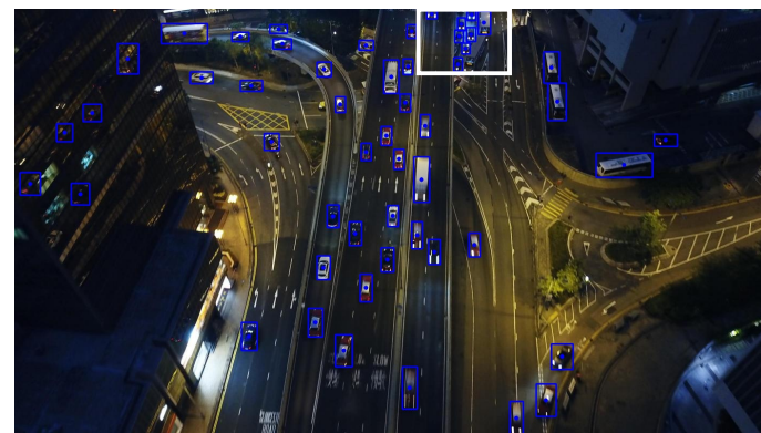
Result (D3F-Det)
