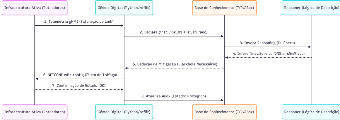
Figure 2: Diagrama de Sequência da Mitigação de DDoS via DT-II
