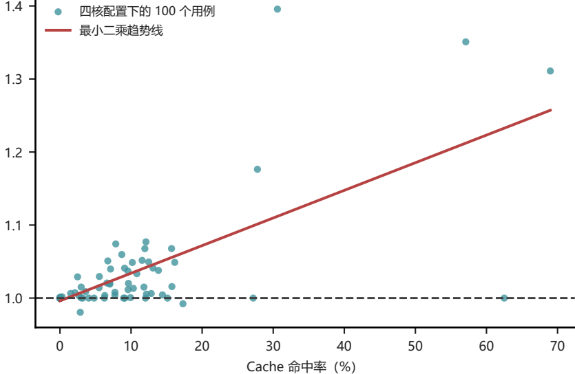
只读 Cache 相对无 L2 的加速比 (倍)
