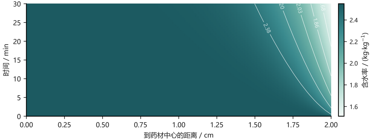
干燥前沿 30 min 内推进到 1.34 cm
