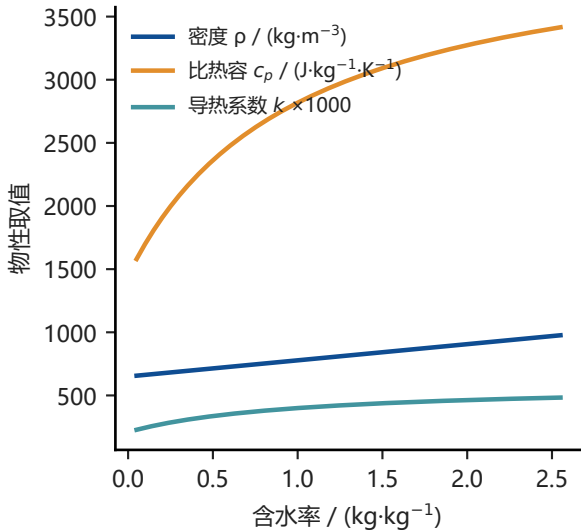
物性随含水率单调增大
