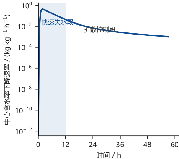
失水速率在 12 h 后转入扩散控制
