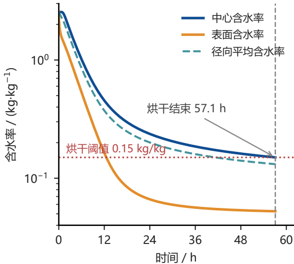
中心含水率是烘干判据的控制点
