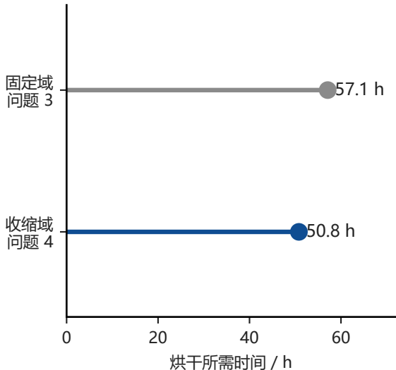
收缩使烘干时间缩短 11.0%
