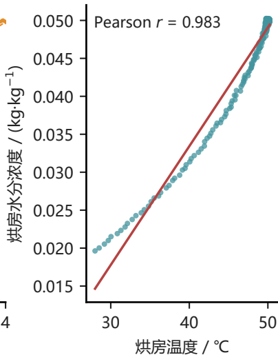
两工况高度线性相关
