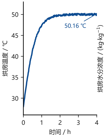
烘房温度在 4 h 内趋稳
