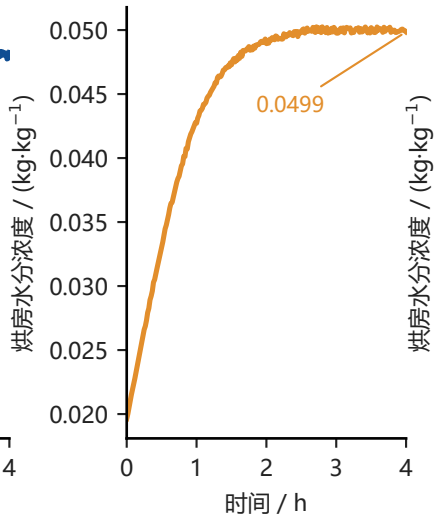
烘房水分浓度同向上升
