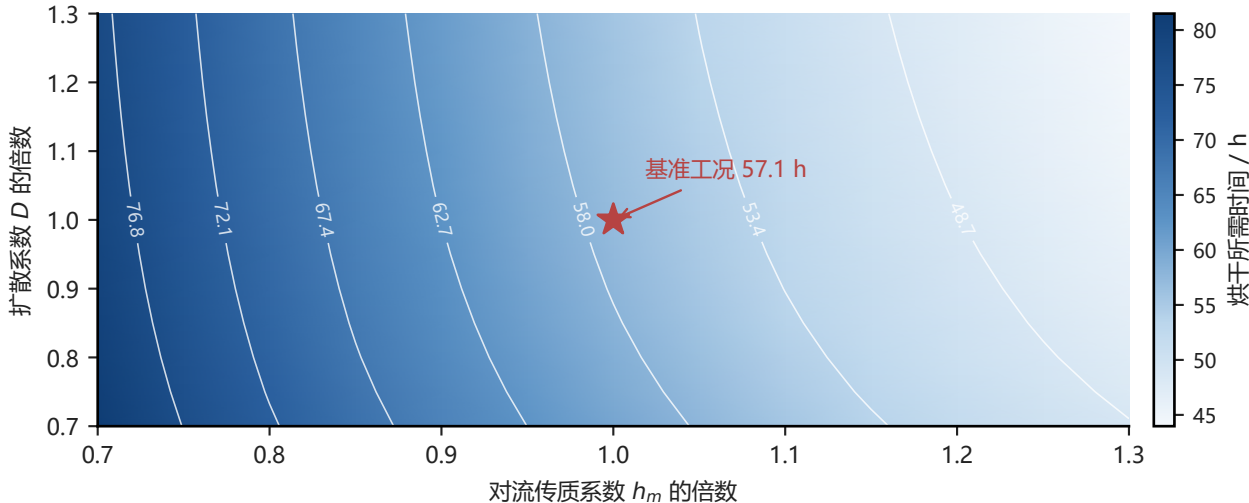
烘干时间对扩散系数与传质系数的二维响应
