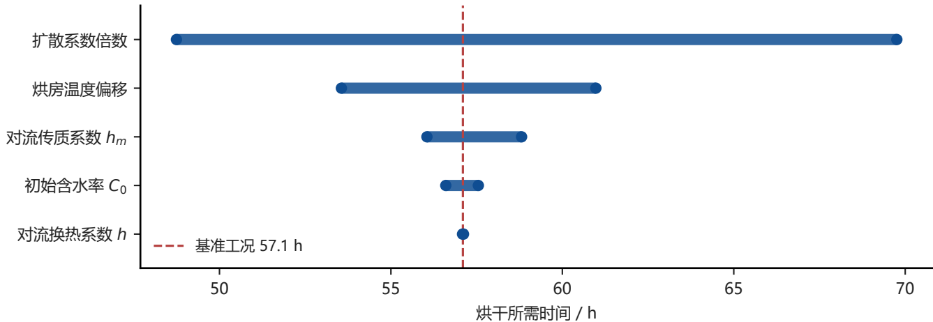
参数 \pm 20\% 扰动下的烘干时间变化
