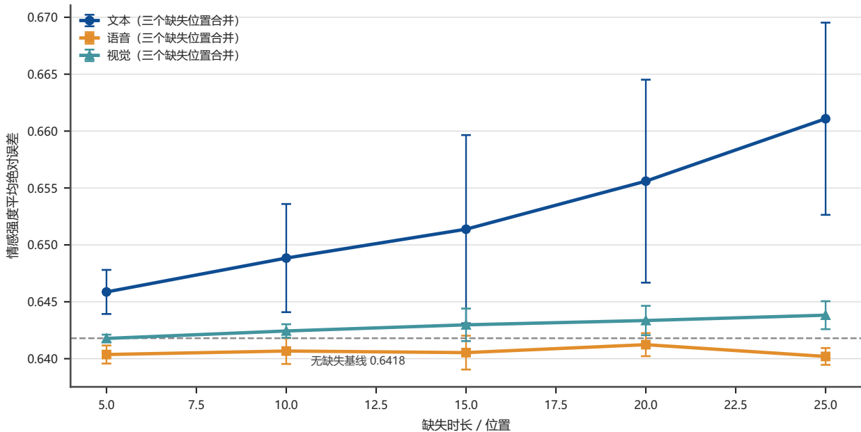
缺失时长对情感强度误差的影响（误差棒为序列前/中/后三个缺失位置的标准差）
