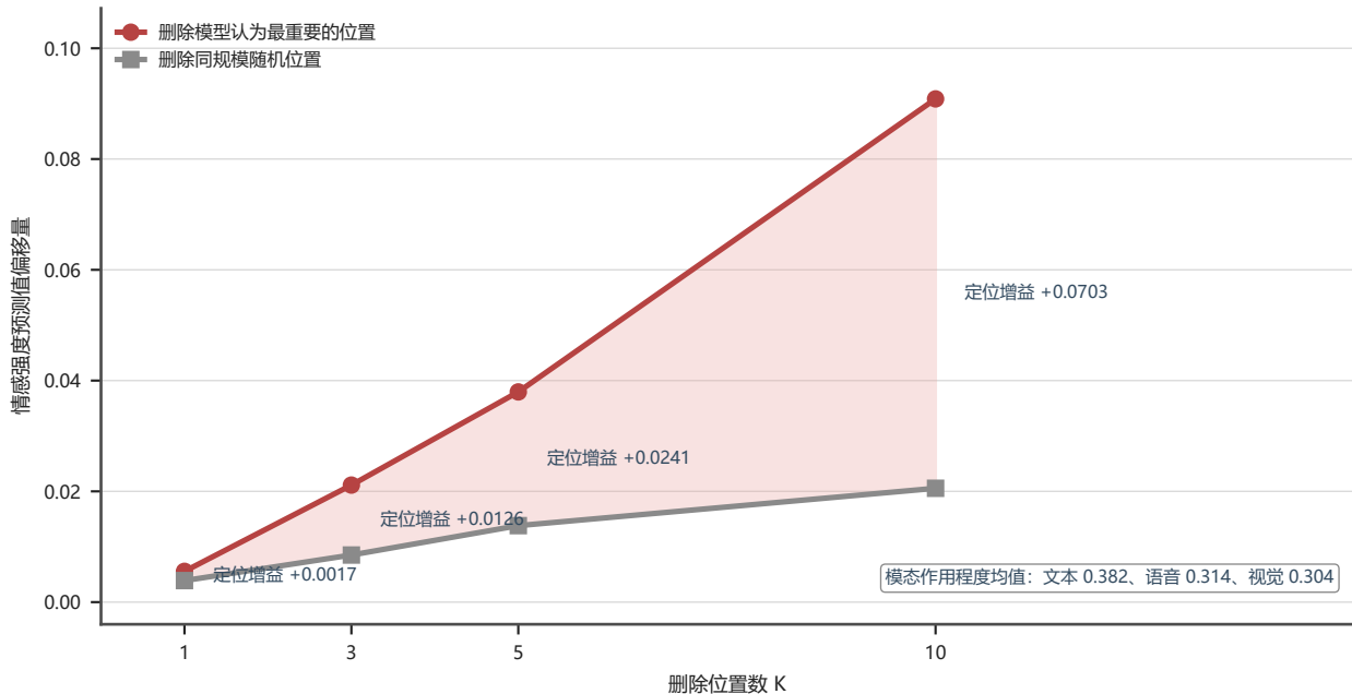
证据定位的删除实验：删除重要位置比删除随机位置引起更大的预测偏移
