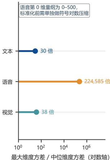
(b) 维度方差量纲差异
