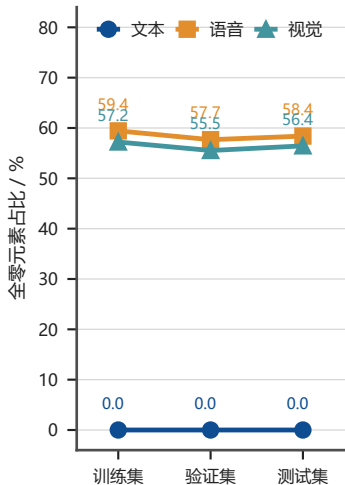
(a) 三模态零值占比
