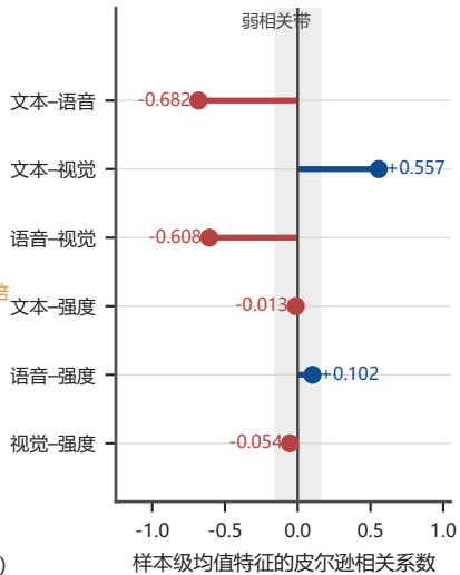
(c) 模态间与模态-强度相关
