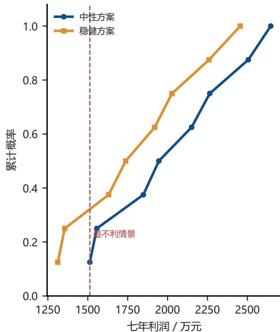
利润的经验累计分布
