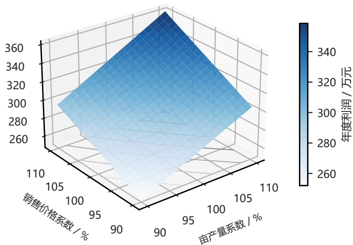
产量与价格双因子响应面
