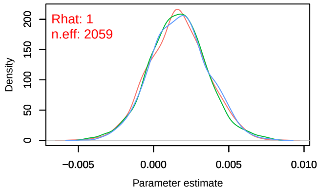
Density – B[chelsa_tas (C4), sp_38 (S38)]
