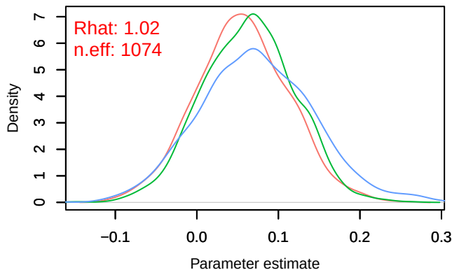
Density – B[chelsa_hurs (C2), sp_5 (S5)]
