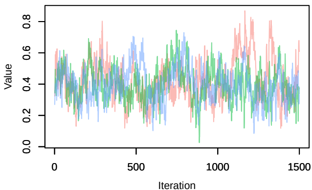
Trace – B[chelsa_hurs (C2), sp_30 (S30)]
