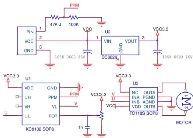
图五 舵机驱动电路
