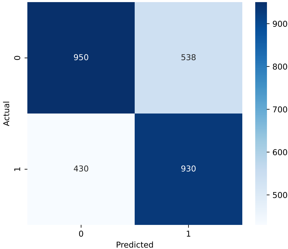
Confusion Matrix: Aktien → GPR, 2001-2021
