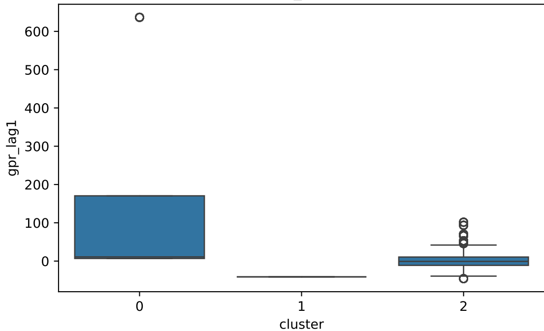
gpr_lag1
