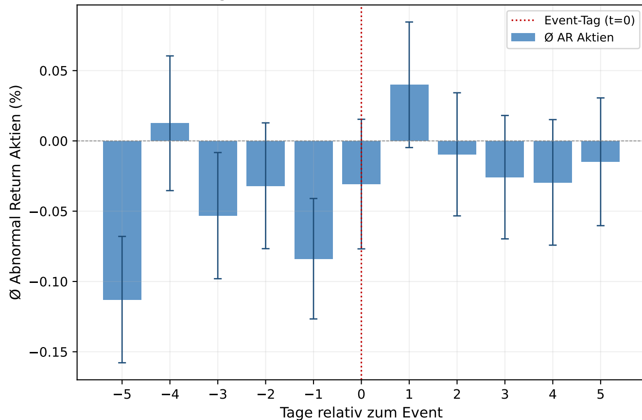
Tägliche durchschnittliche AR ( \pm 95\% KI)
