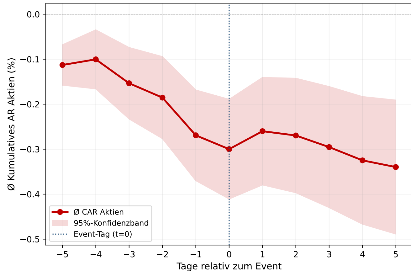
Kumuliertes CAR im Ereignisfenster
