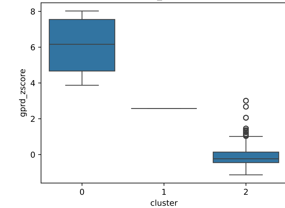
gprd_zscore
