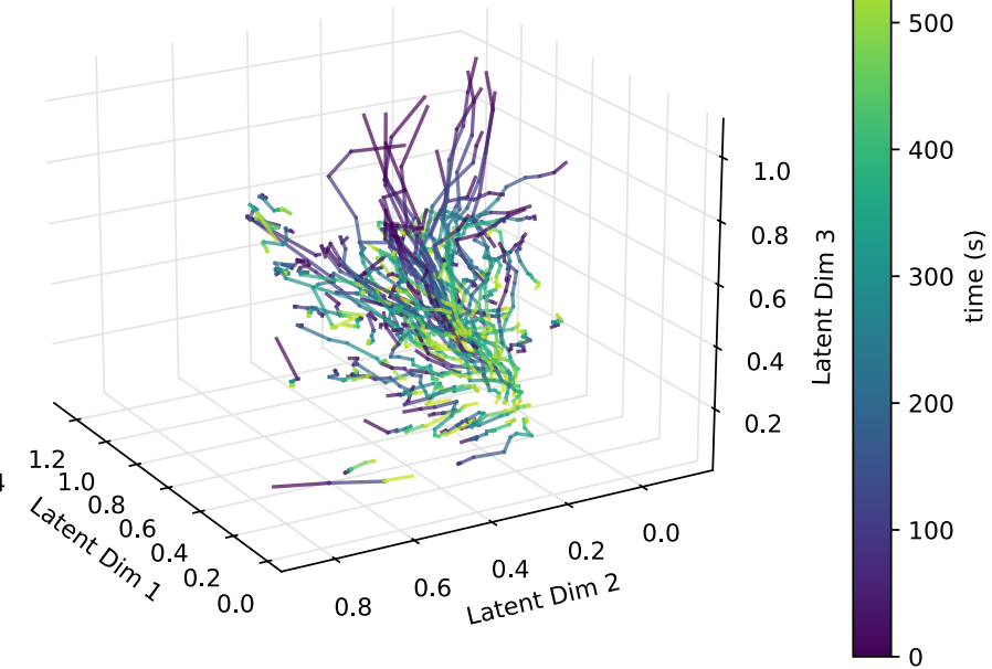
c) Autoregressive (AR)
