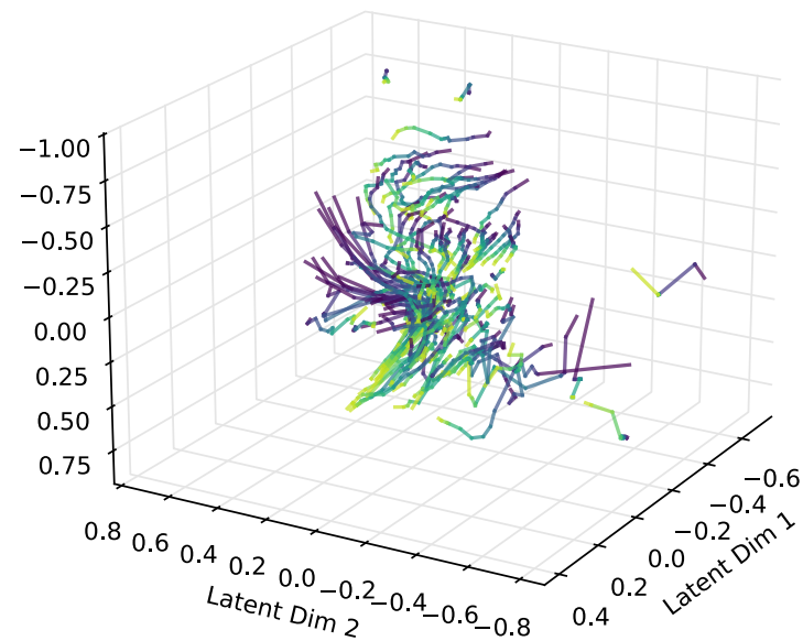
a) SINDy
