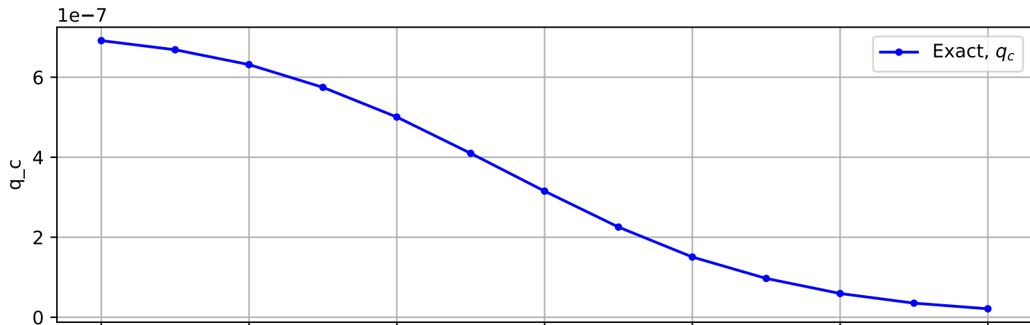
Trajectory No. 1045
