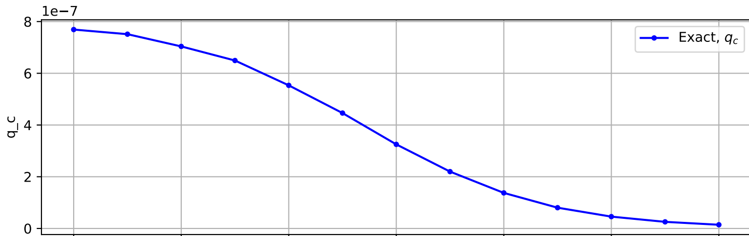
Trajectory No. 1093
