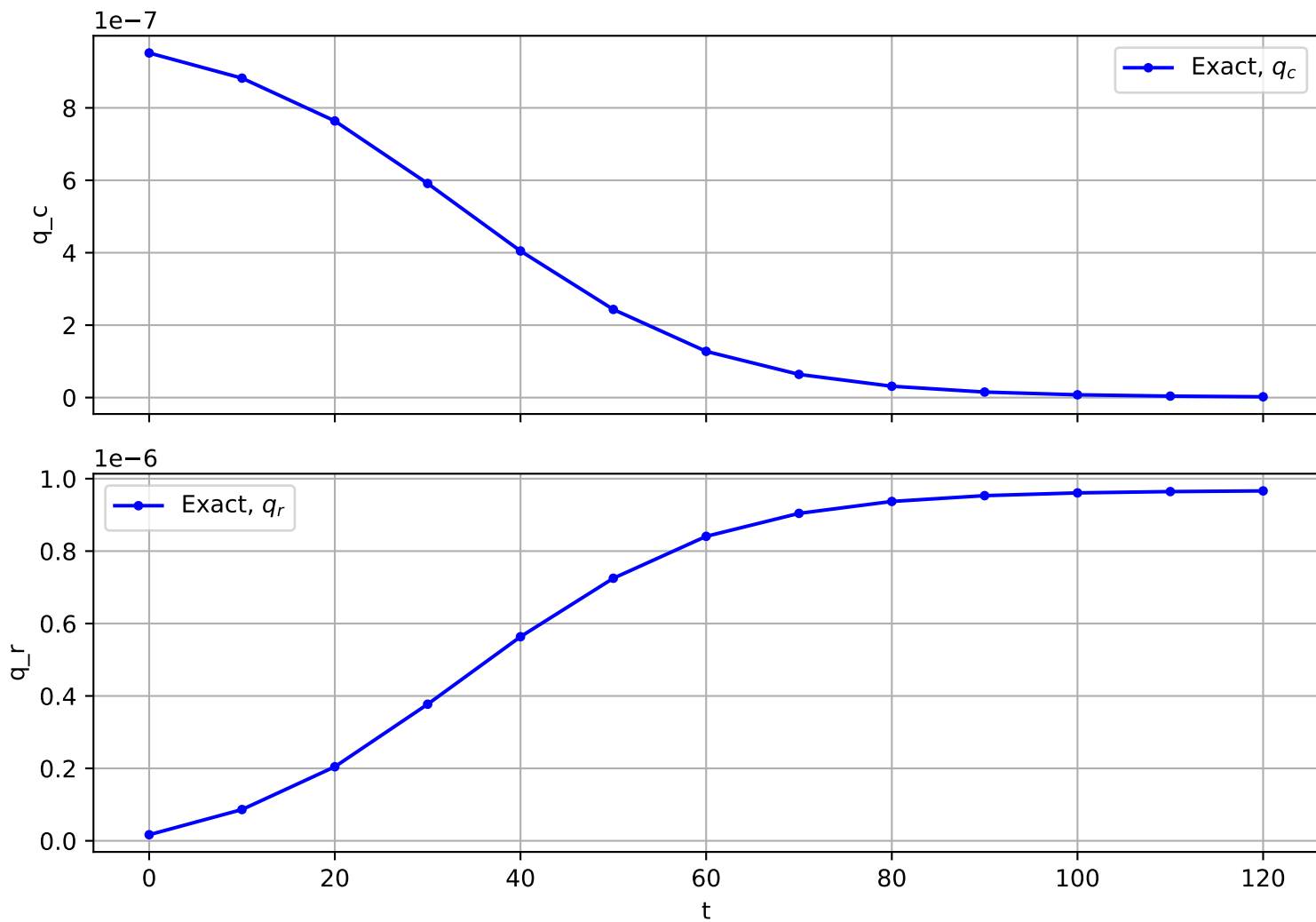
Trajectory No. 1173
