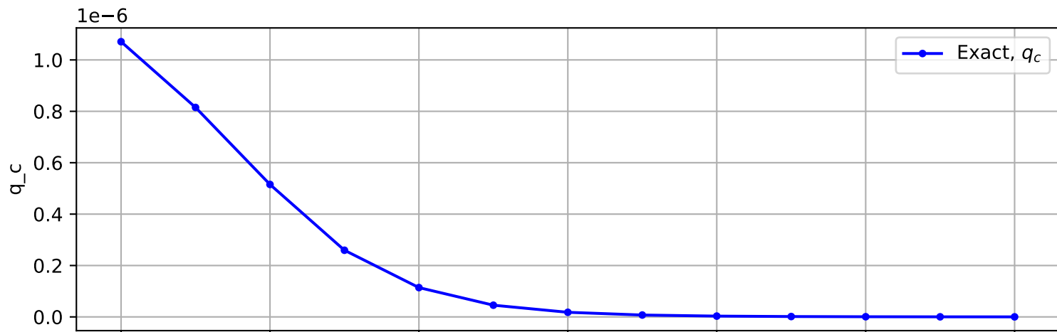
Trajectory No. 1187
