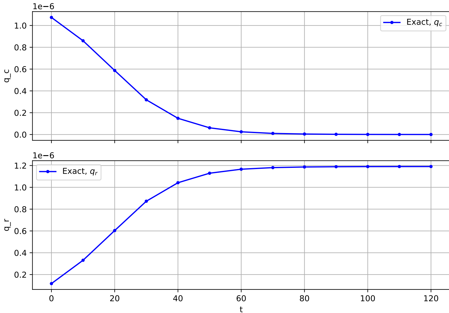
Trajectory No. 1201
