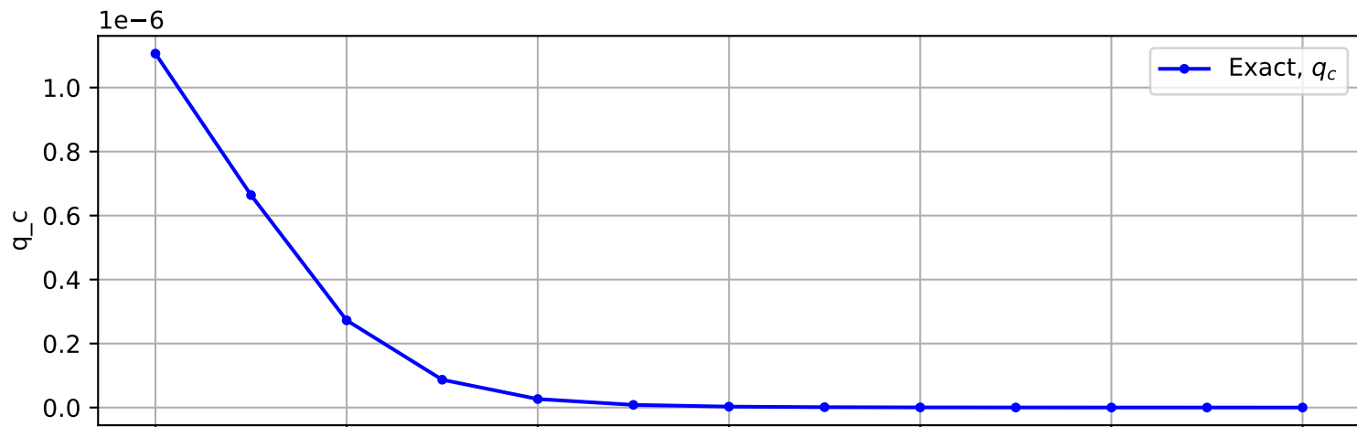
Trajectory No. 1220
