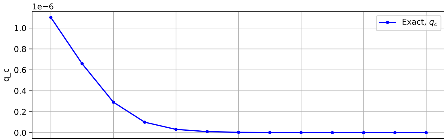
Trajectory No. 1222
