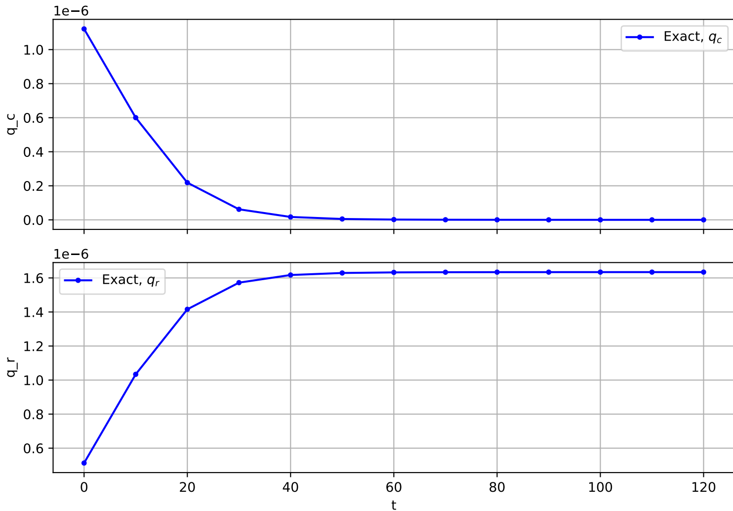
Trajectory No. 1258
