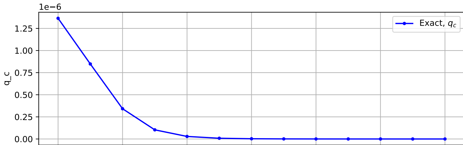
Trajectory No. 1279
