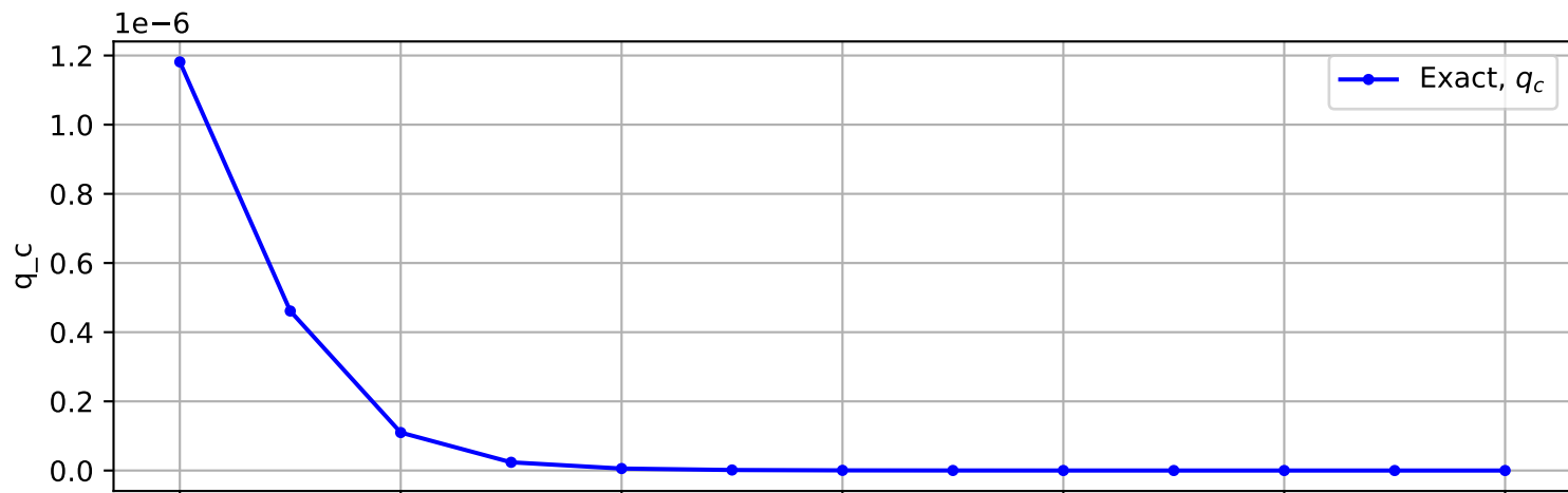
Trajectory No. 1307
