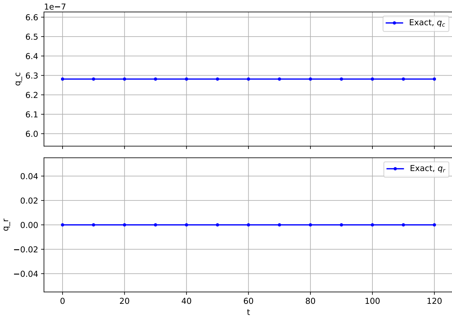
Trajectory No. 1353
