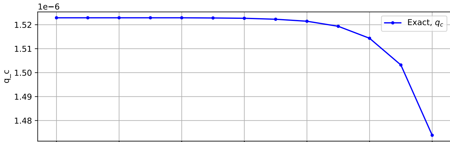
Trajectory No. 1407
