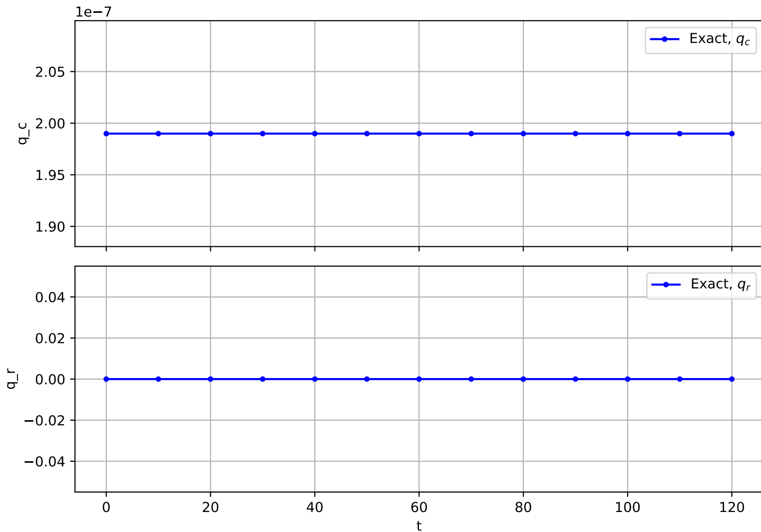
Trajectory No. 1449
