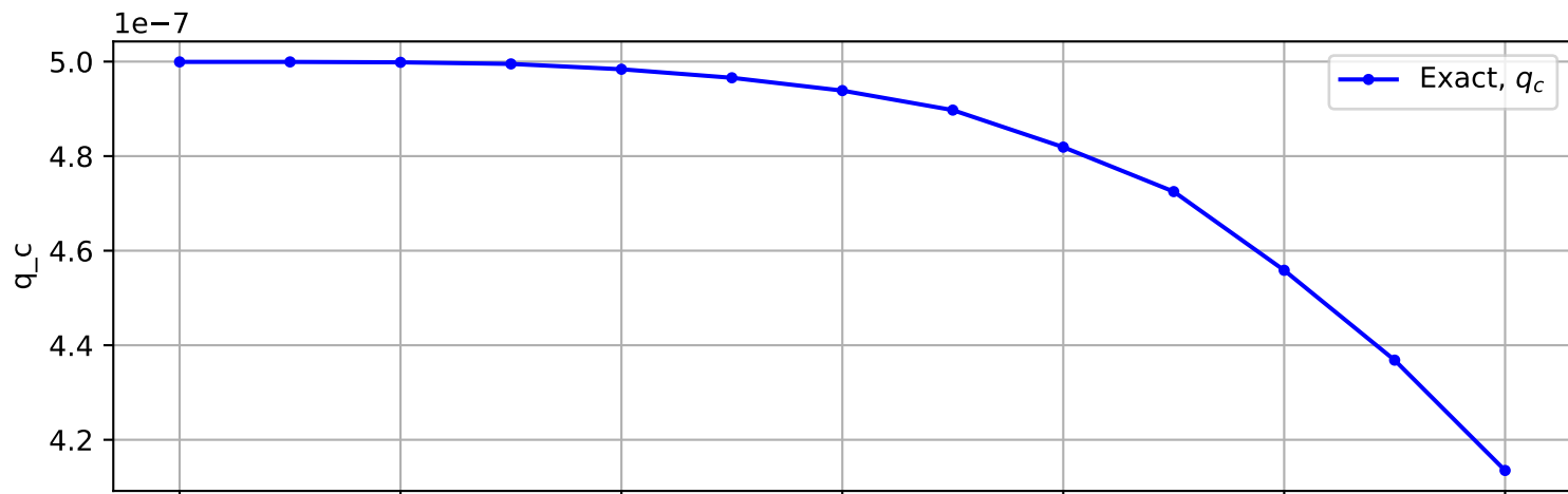
Trajectory No. 1488
