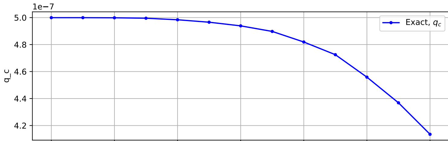
Trajectory No. 1489
