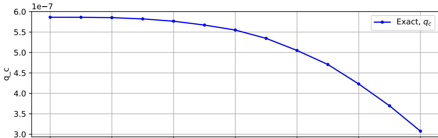
Trajectory No. 1503
