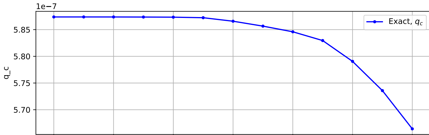
Trajectory No. 1523
