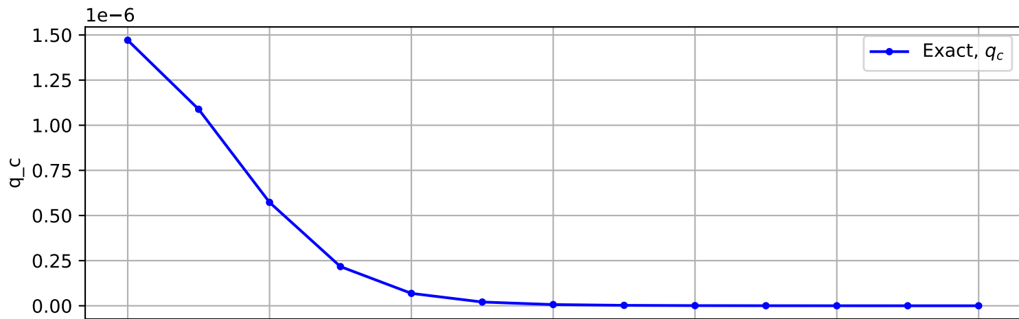
Trajectory No. 1748
