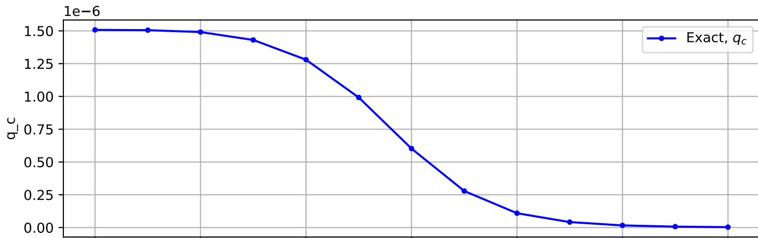
Trajectory No. 183
