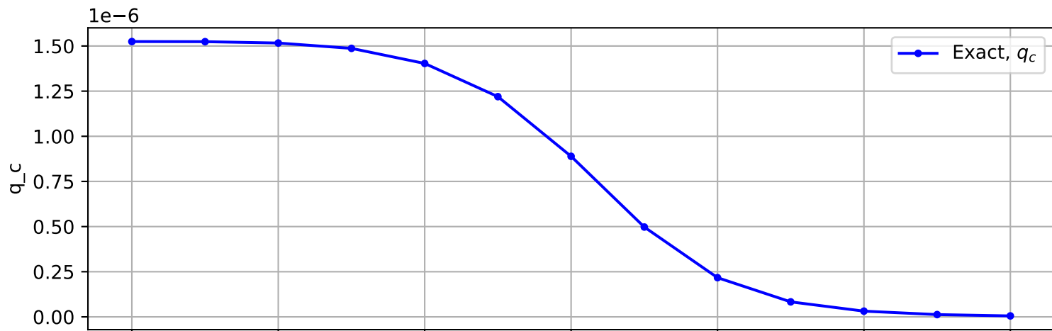
Trajectory No. 191
