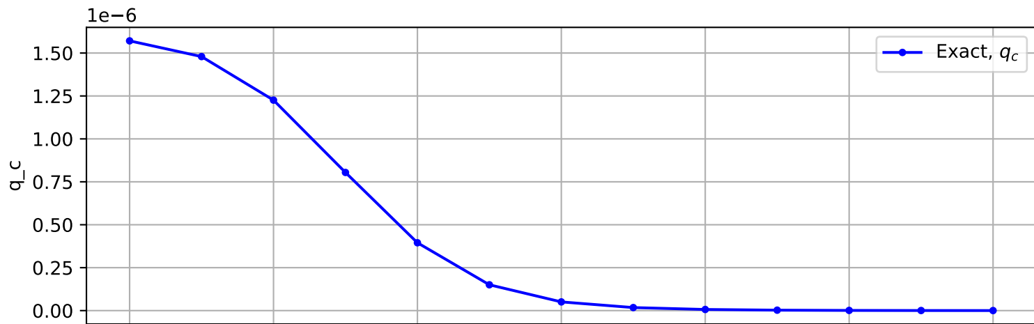
Trajectory No. 213
