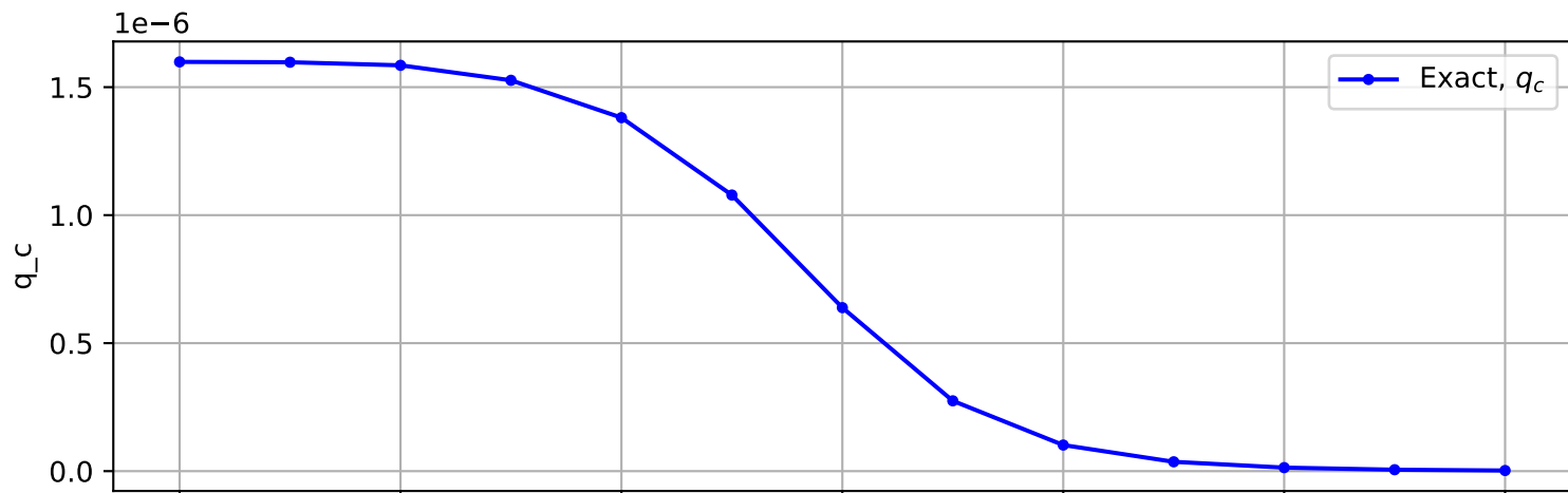
Trajectory No. 228
