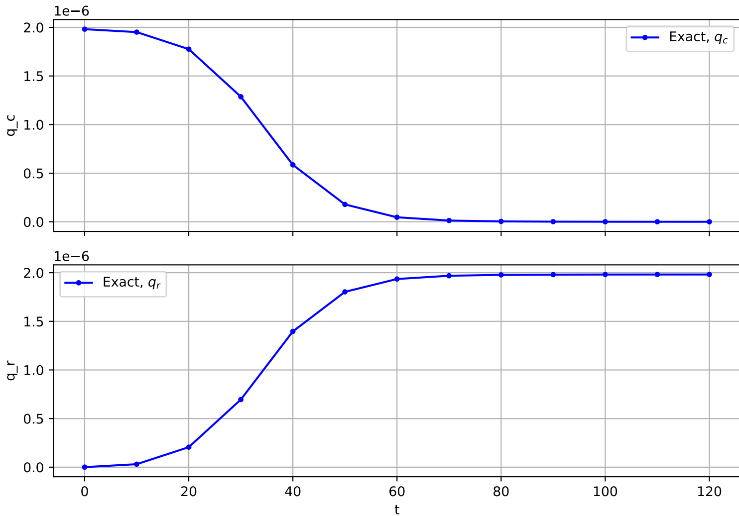
Trajectory No. 264
