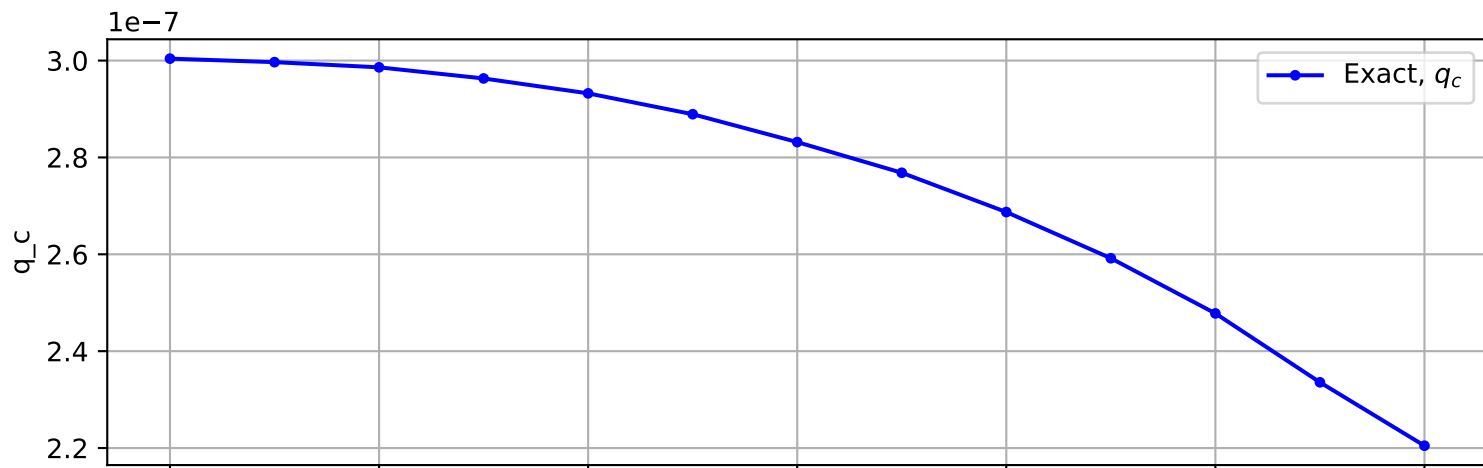
Trajectory No. 305
