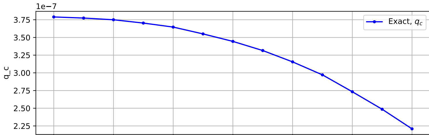
Trajectory No. 362
